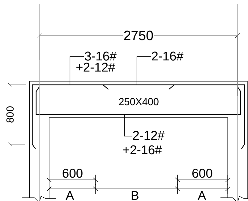
S.R.B.-E5,E6/C5,C6 BEAM SIZE- 250X400
