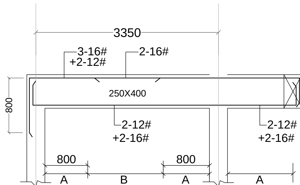
S.R.B.- E5,C5/E6,C6 BEAM SIZE- 250X400
